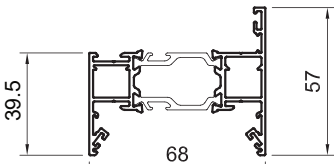
SPW716717G SPW716717W SPW716717DWG deep outerframe
